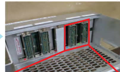
コネクタ受け（左：正常、右：ピン曲げ）
